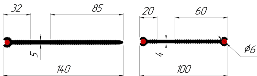
Гидрошпонка ТПС-140-1
